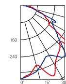
Прозрачный рассеиватель
